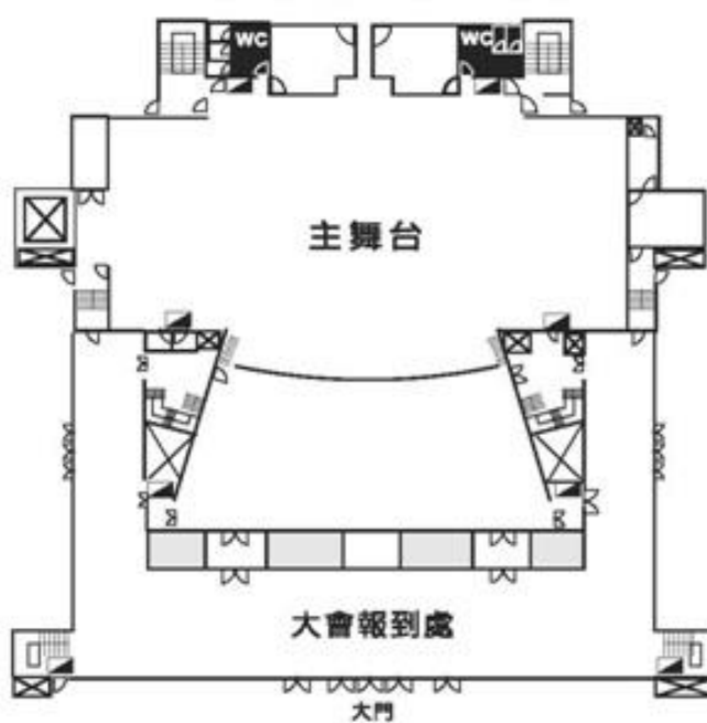
逸仙館一樓平面圖 Sun Yat-sen Floor Plan
